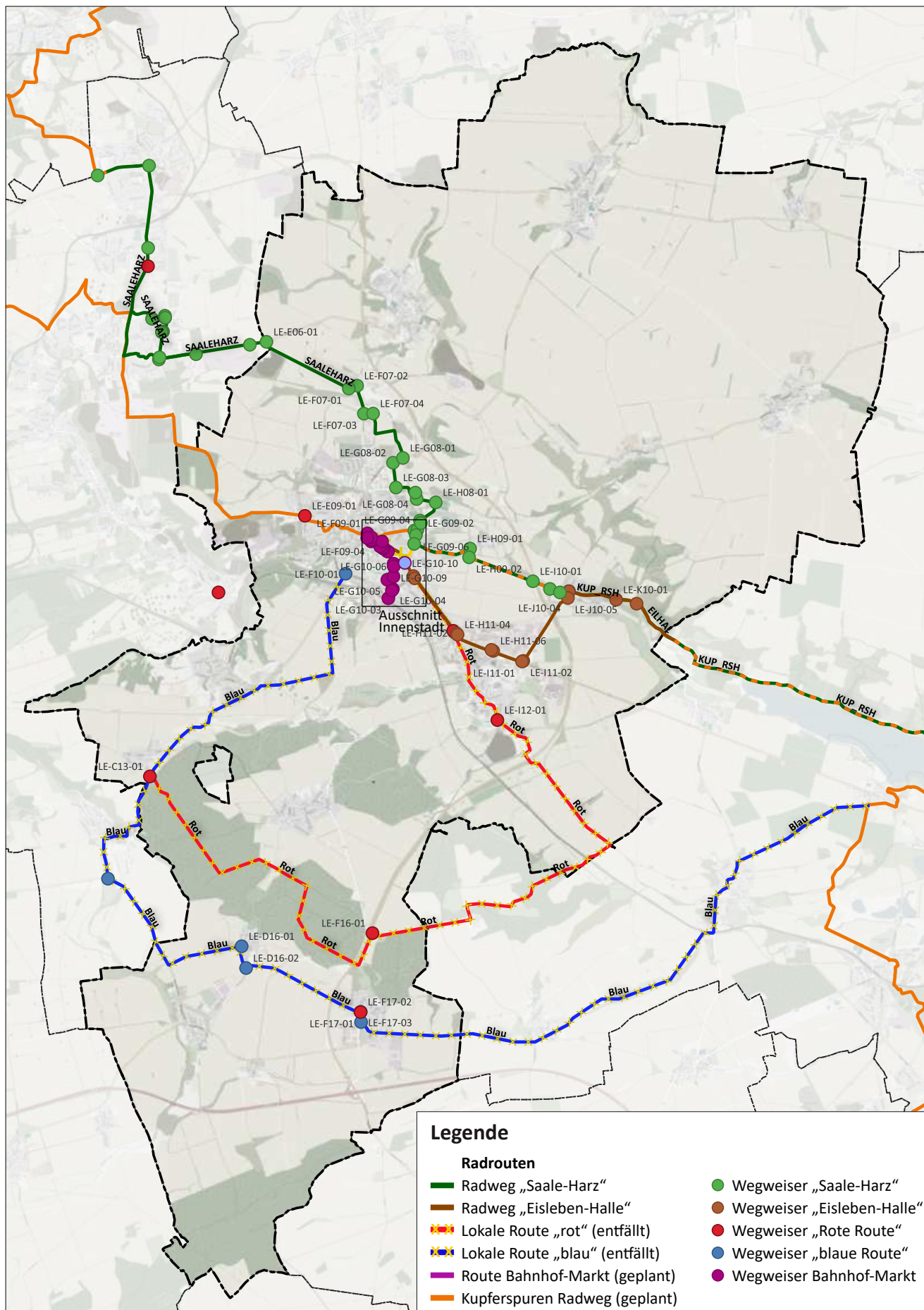
Abb. 7 Übersicht bestehende und geplante Radrouten mit Wegweisern
